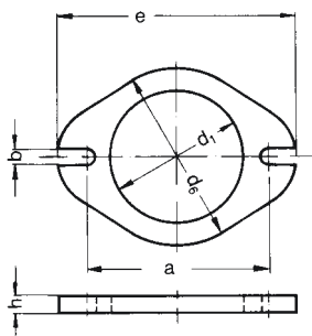
Schweißflansch für saugseitige Anschlußrohrleitung Welding flange for pipe connection on intake side
